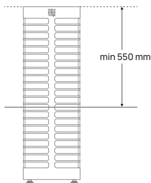
Рисунок 2. Установка каменки HUUM STEEL, частично погруженной в полоч.
